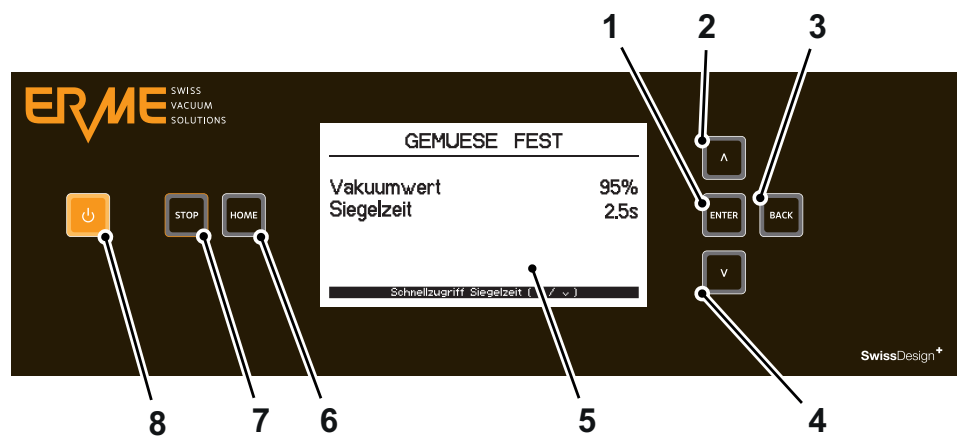
Abb. 5: Bedienpanel
