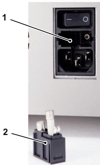
Abb. 18: Sicherung
